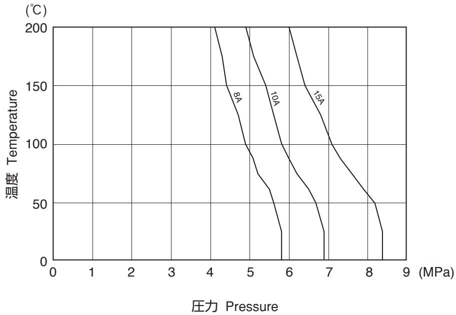
小口径クランプ Small Dia. Clamp (CP2K) Nom.Size 8A, 10A, 15A
