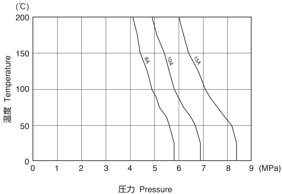
小口径2Dクランプ Small Dia. 2D-Clamp (CP2D) Nom.Size 8A, 10A, 15A
